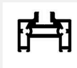
SWING DOOR HORIZONTAL
